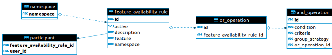
Slika 8 Shema baze za feature flags servis
