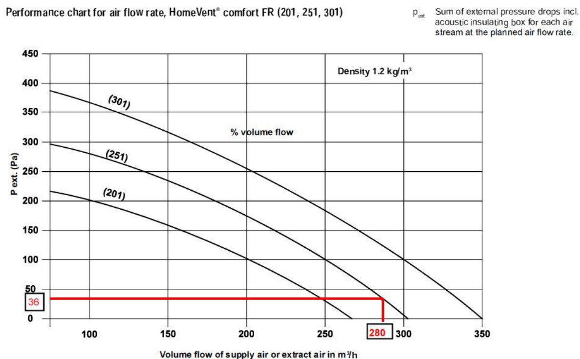
Slika 3.24 - Prikaz karakteristike rada uređaja, protok zraka u ovisnosti o padu tlaka [4]
