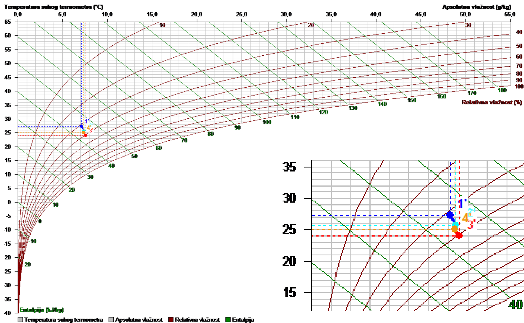
Slika 5.12 - Prikaz druge točke drugog mjerenja u Mollierovom dijagram [13]
