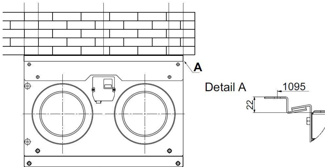
Slika 3.26 - Montaža uređaja na strop [4]
