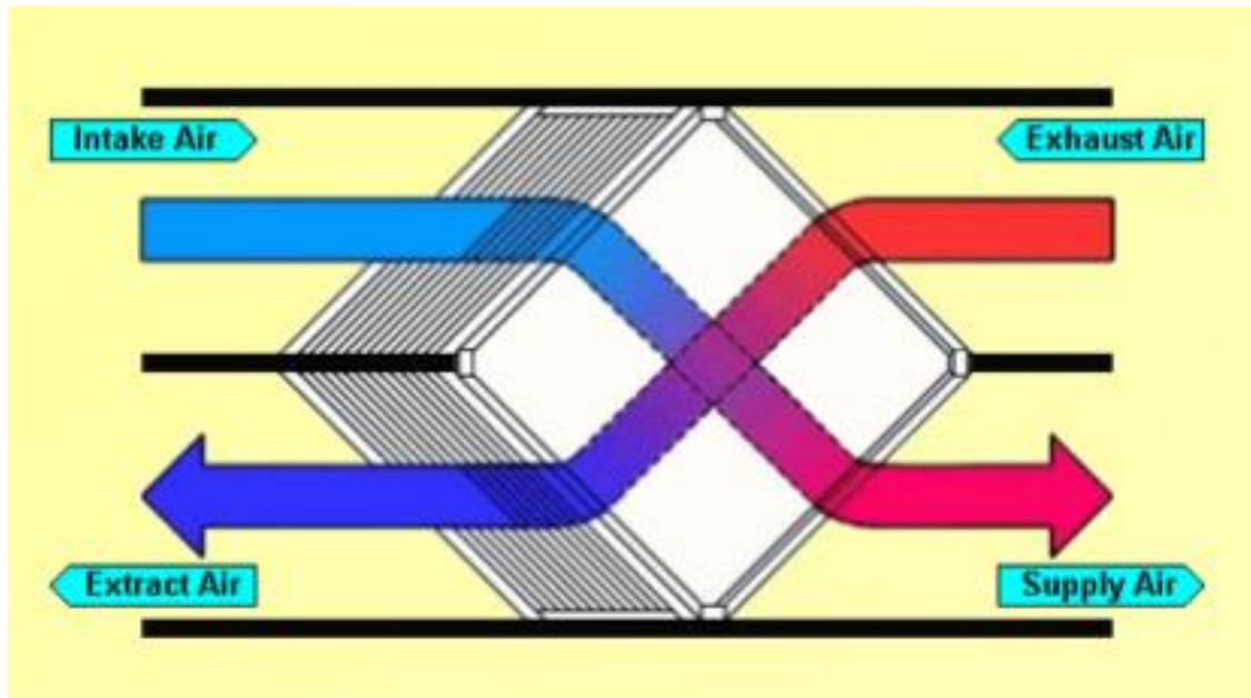
Slika 2.2 - Prikaz principa rada rekuperatora [5]
