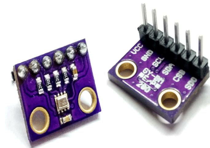
Slika 4.4. BMP280 senzor [17]
