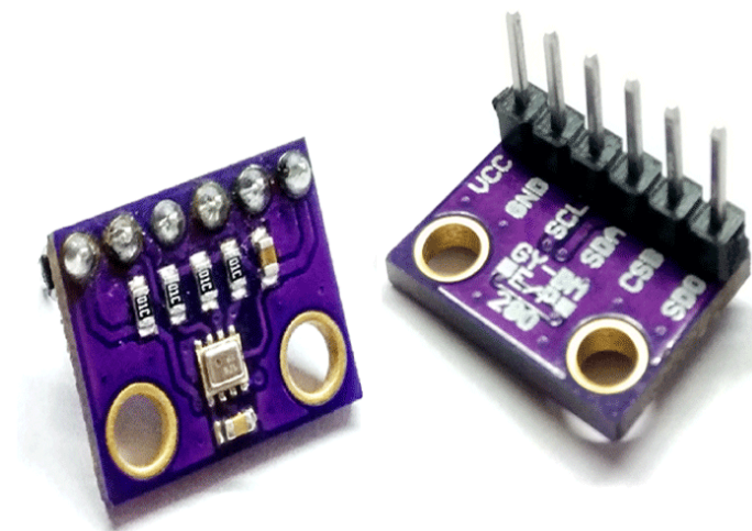
Slika 4.4. BMP280 senzor [17]
