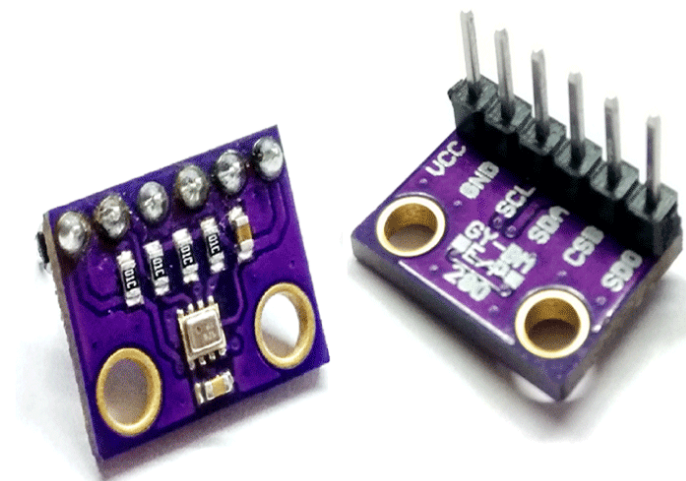
Slika 4.4. BMP280 senzor [17]
