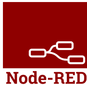
Slika 4 - Node-RED logotip
