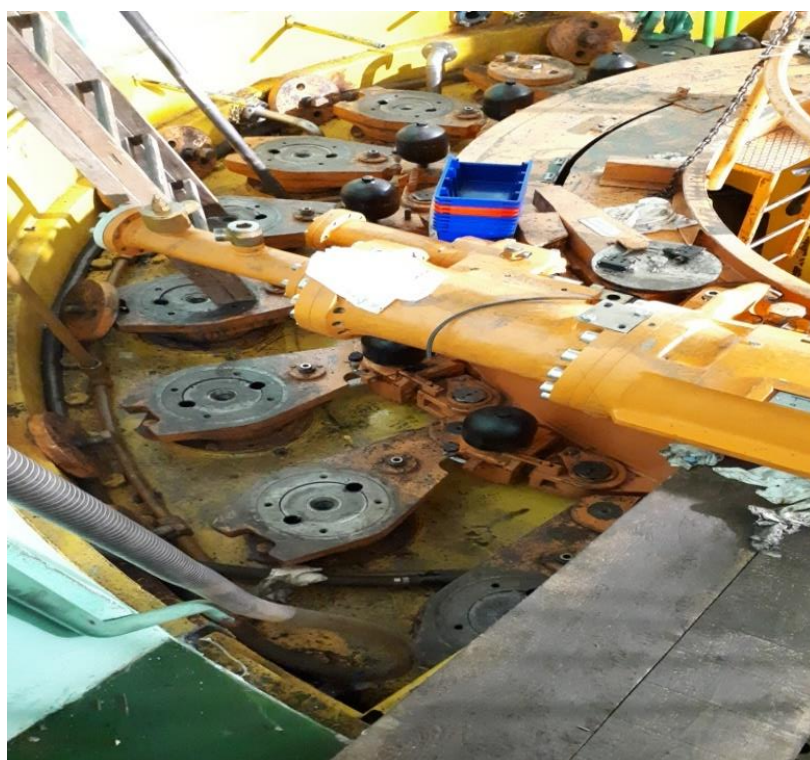
Slika 4. 24. Hidraulički mehanizam lopatica [15]
