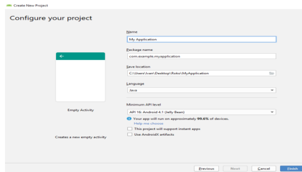
Slika 21: Konfiguriranje projekta
