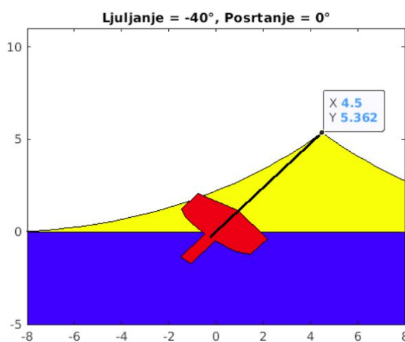
Slika 5.5. Model zaštitne zone jedrilice za kut ljuljanja \alpha različit od 0^\circ
