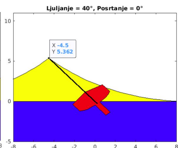
Slika 5.5. Model zaštitne zone jedrilice za kut ljuljanja \alpha različit od 0^\circ
