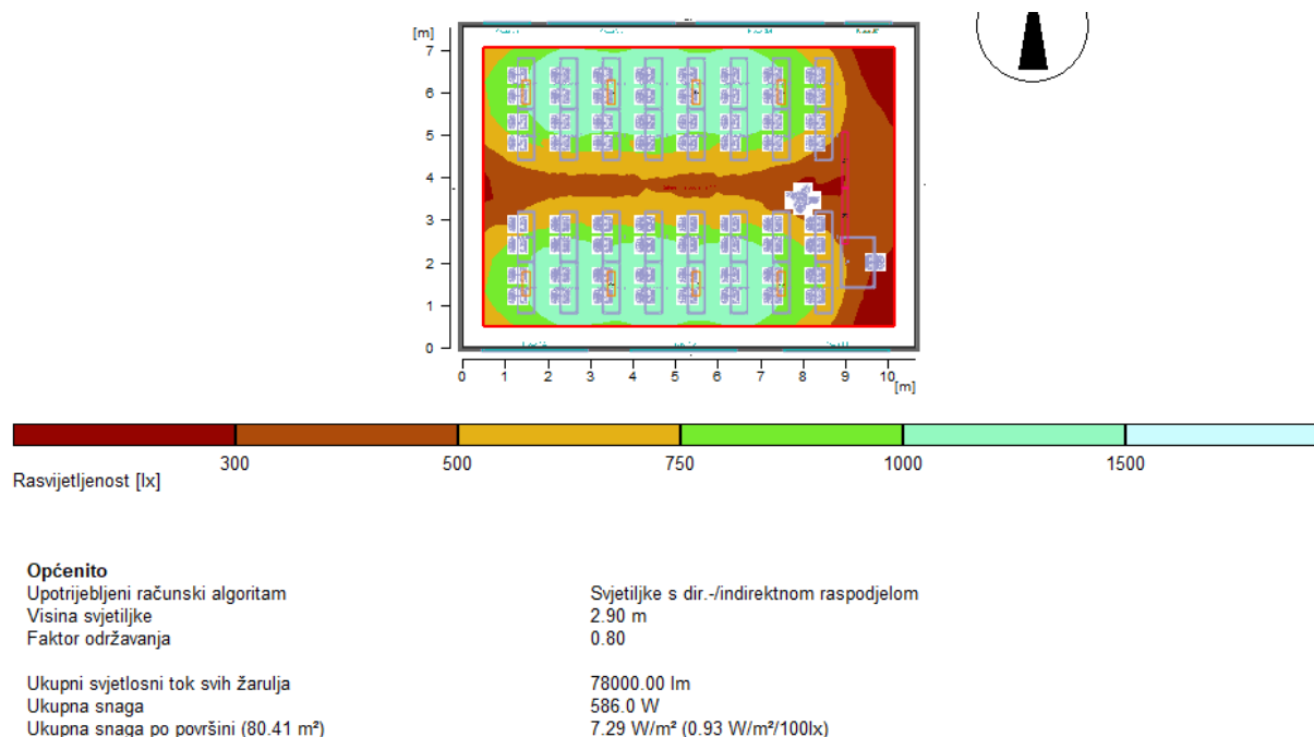
Slika 31. Rezultati proračuna novo projektiranog stanja predavaonice 106
