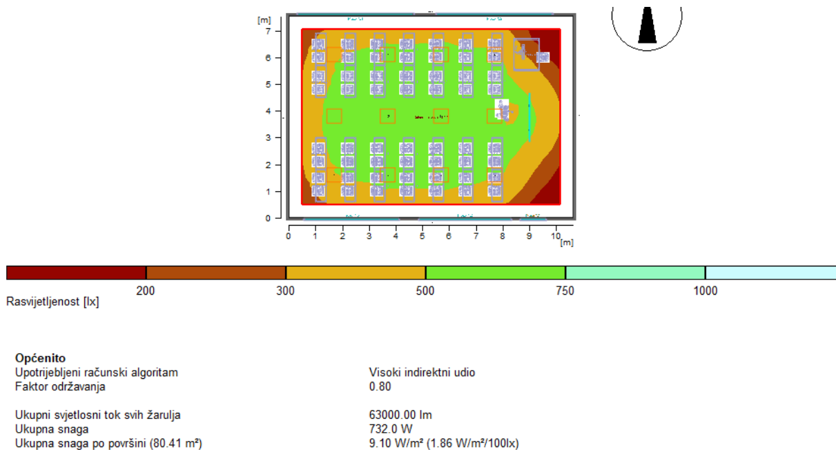
Slika 18. Rezultati proračuna postojećeg stanja predavaonice 102
