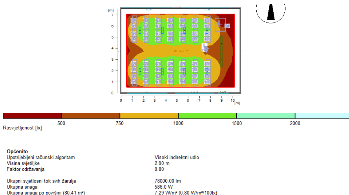
Slika 25. Rezultati proračuna novo projektiranog stanja predavaonice 104
