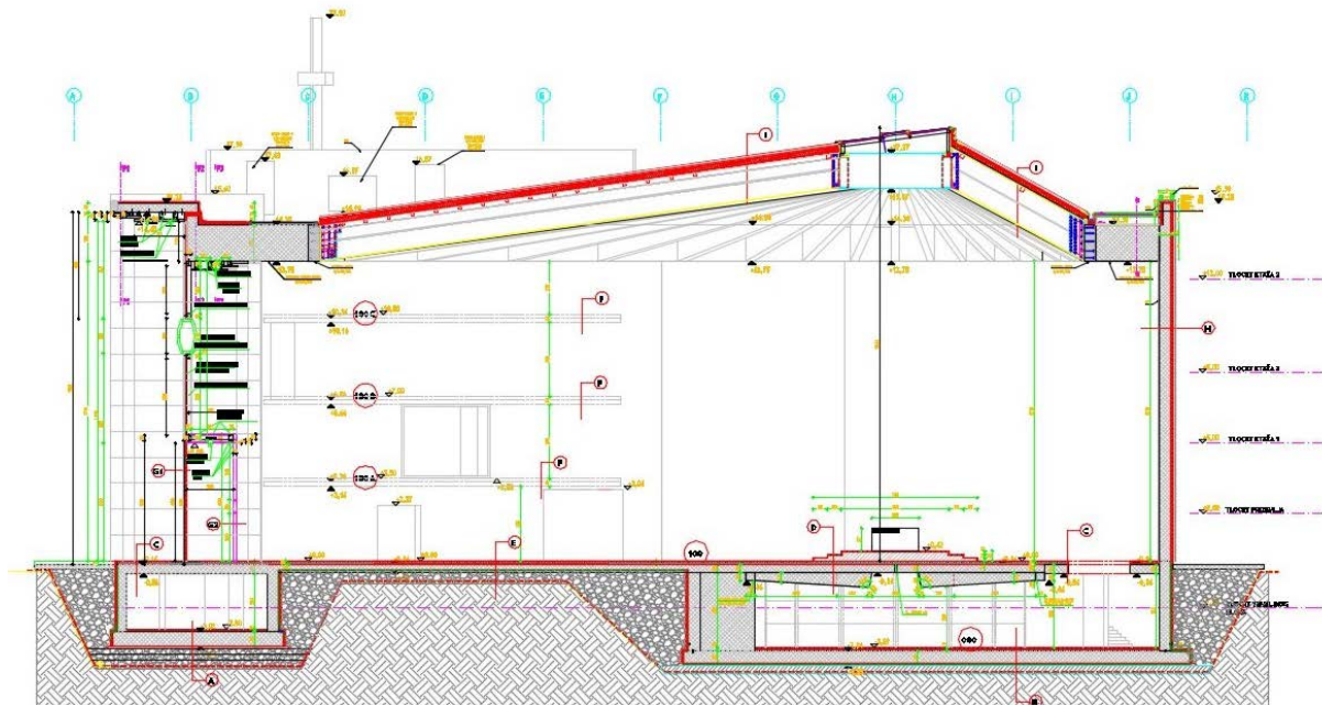
Slika 1.3 - Presjek bazilike u Solinu (presjek preuzet iz glavnog projekta) [1]
