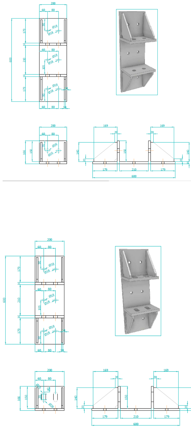
Slika 7.8 - Oslonci glavnih nosača 2,3,4 [2]
