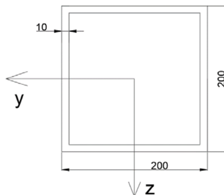
Slika 6.10 - Dimenzije presjeka profila glavnog nosača
