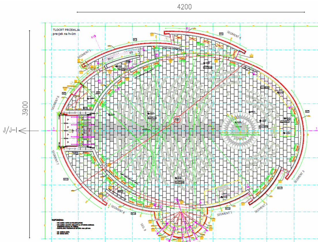
Slika 1.2 - Tlocrt bazilike u Solinu (tlocrt preuzet iz glavnog projekta) [1]
