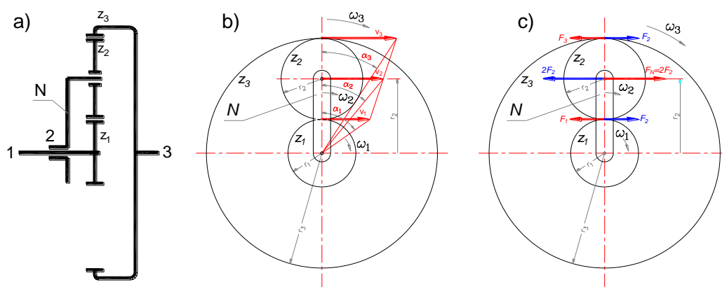
Slika 3.21 - Planetarni prijenosnik
