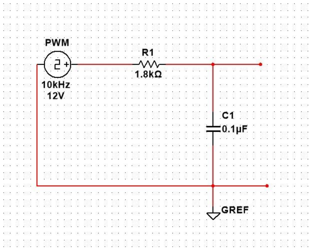
Slika 3.4. Korišteni RC filter
