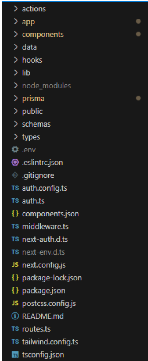
Slika 2: Struktura projekta.
