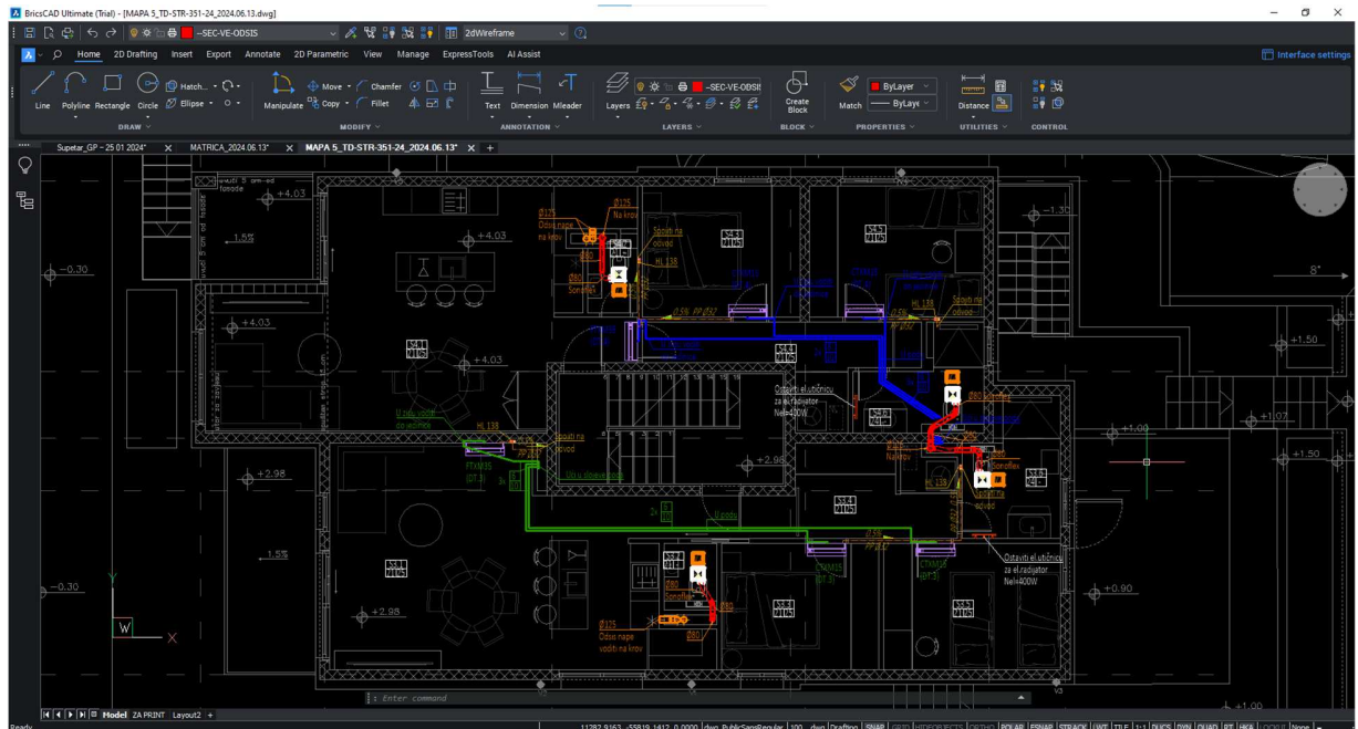
Slika 4.21-Tlocrt kata sa svim instalacijama
