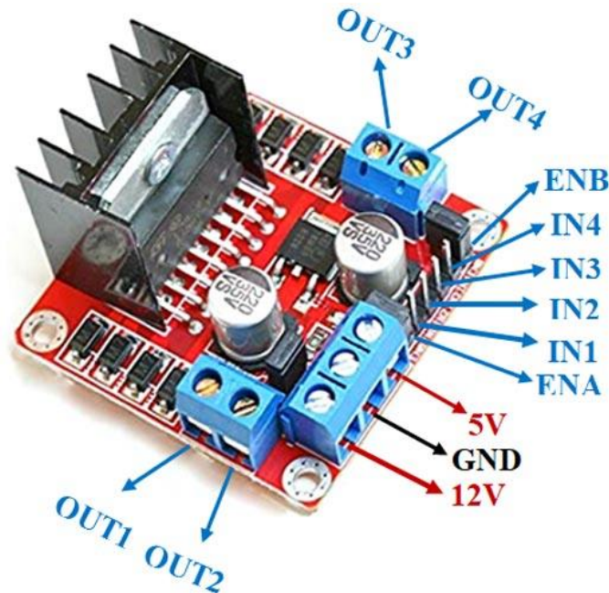
Slika 9. L298N modul [11]
