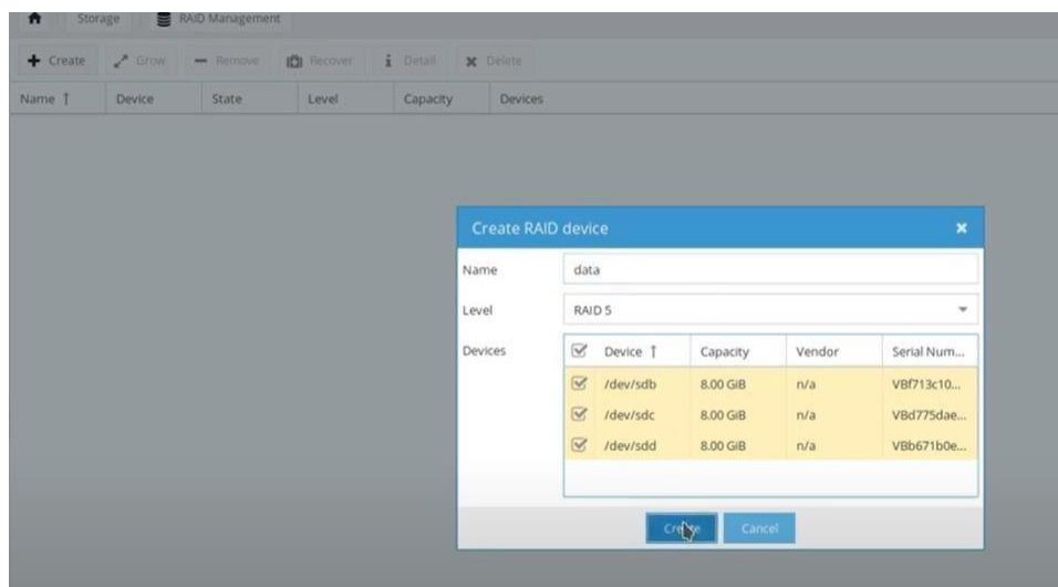
Slika 9.16 RAID 5 konfiguracija
