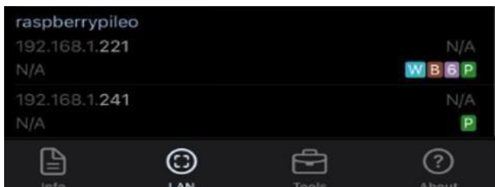
Slika 8.8 NetAnalyzer
