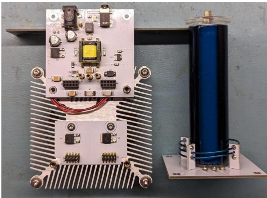
Slika 5. 3: Komponente sustava
