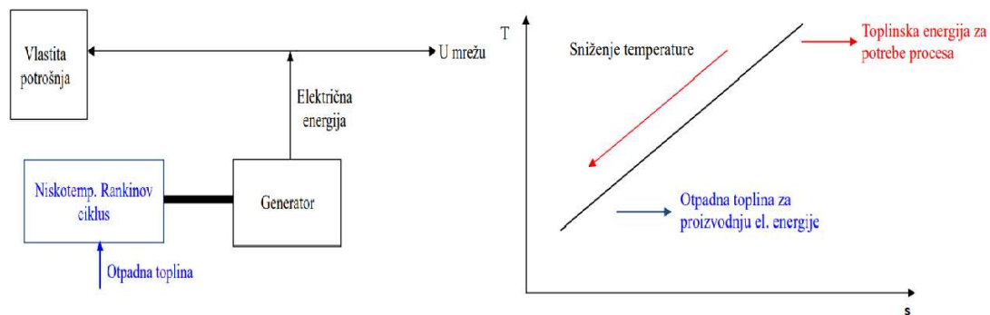
Slika 3.10. "Bottom cycle" kogeneracijsko postrojenje
