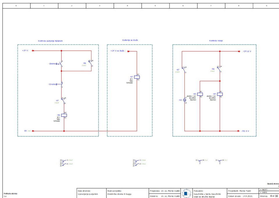
Slika 5.1. Shema kontrole punjenja
