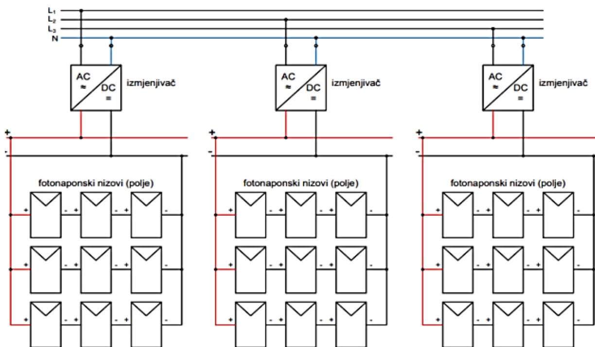
Slika 4.5. Izvedba fotonaponske elektrane koja ima više izmjenjivača [20]
