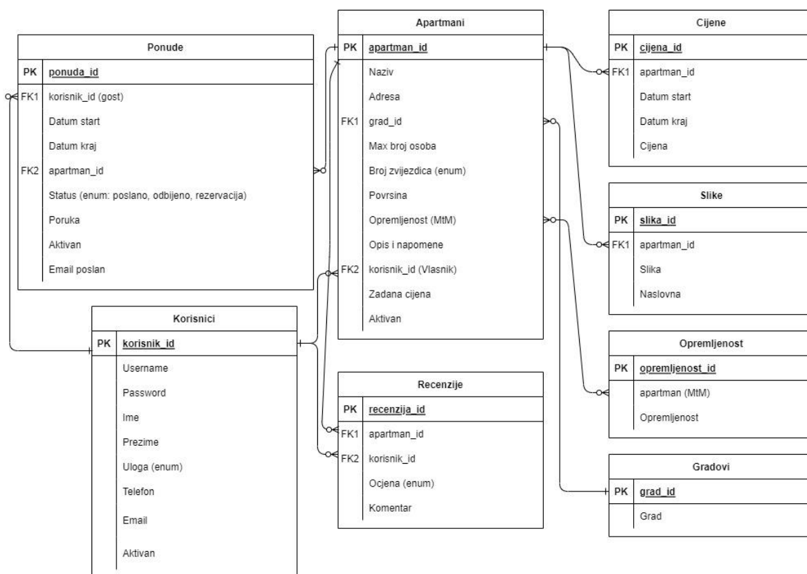
Slika 1 - Baza podataka
