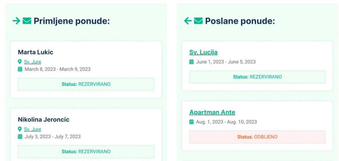
Slika 9 - Upiti
