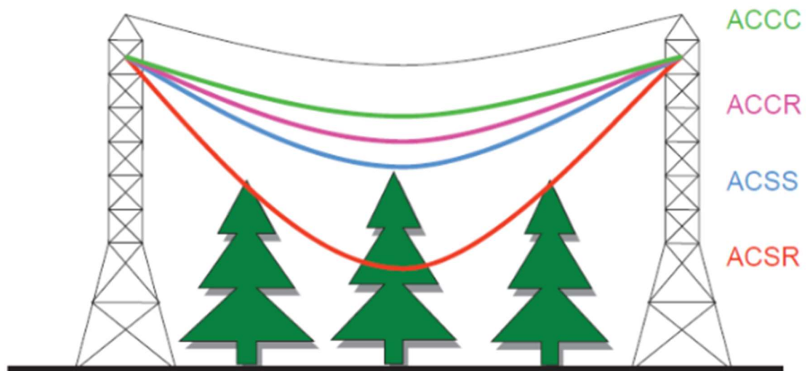
Slika 3.6. Usporedni prikaz provjesa nekih tipova HTLS vodiča u odnosu na klasični ACSR vodič pri temperaturi vodiča od 180 °C [8]
