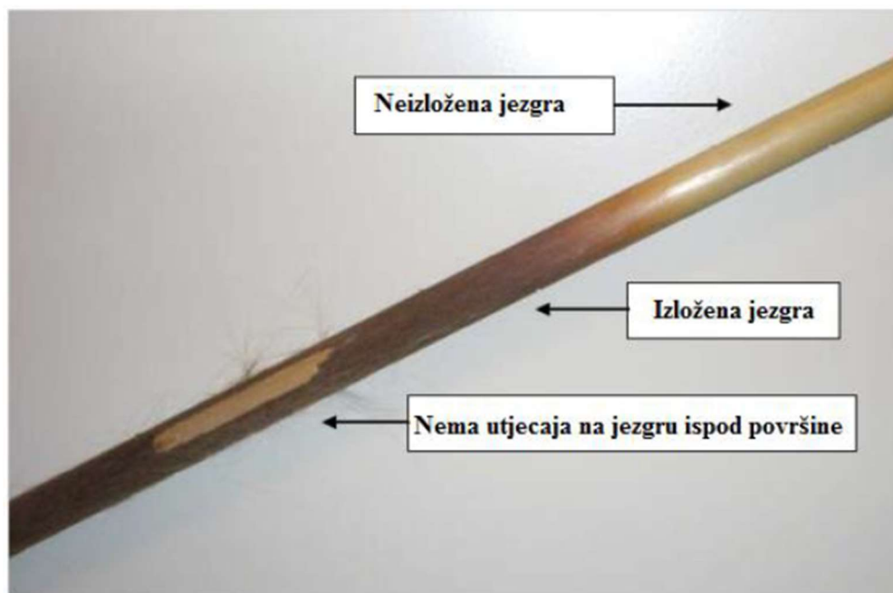
Slika 4.6. Kompozitna jezgra ACCC vodiča nakon izloženosti temperaturi od 220^{\circ}\text{C} 52 tjedna [10]
