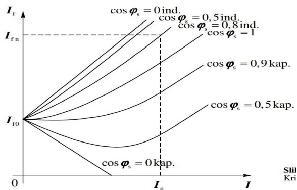
Slika 2.9. Krivulje regulacije [1]
