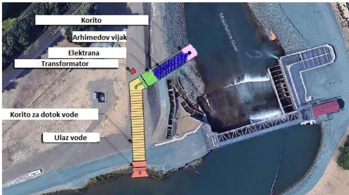
Slika 8.1– Izvedba s betonskim kanalom za dotok vode do turbine [9]
