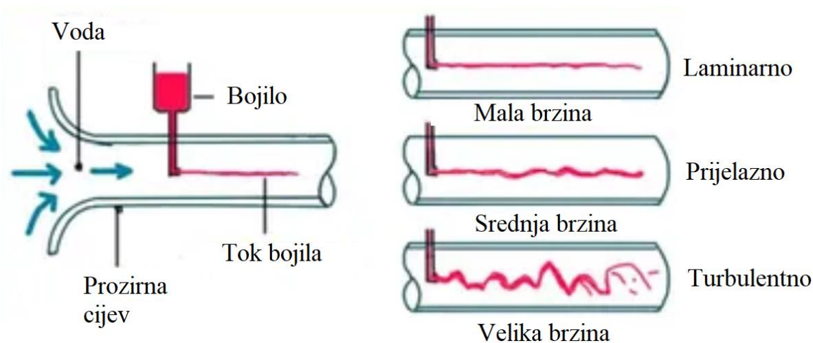
Slika 2.2 – Vrsta strujanja u odnosu na brzinu protoka [4]
