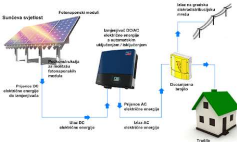
Slika 4.3. Fotonaponski sustav [16]
