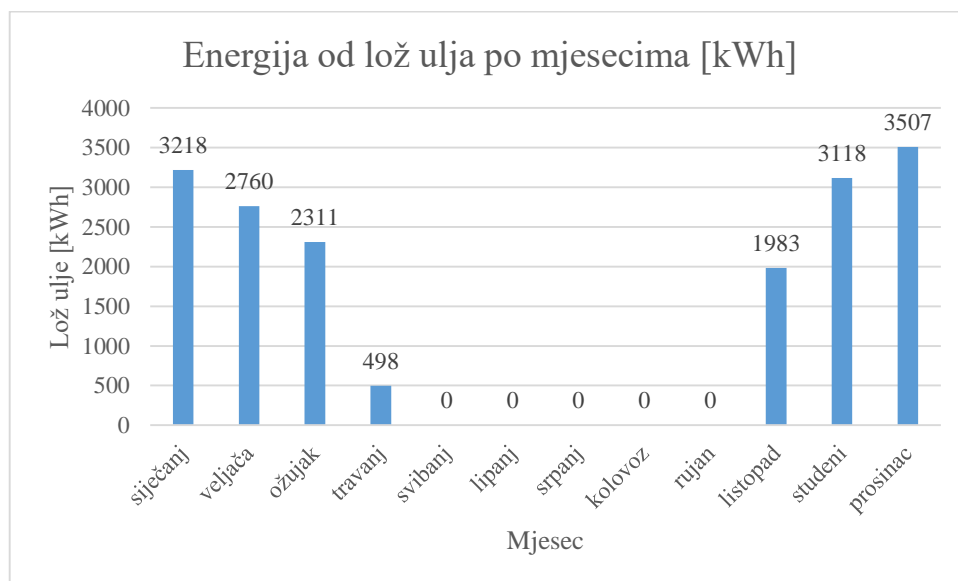
Slika 5.6 - Potrošnja lož ulja u kilovat satima [kWh]
