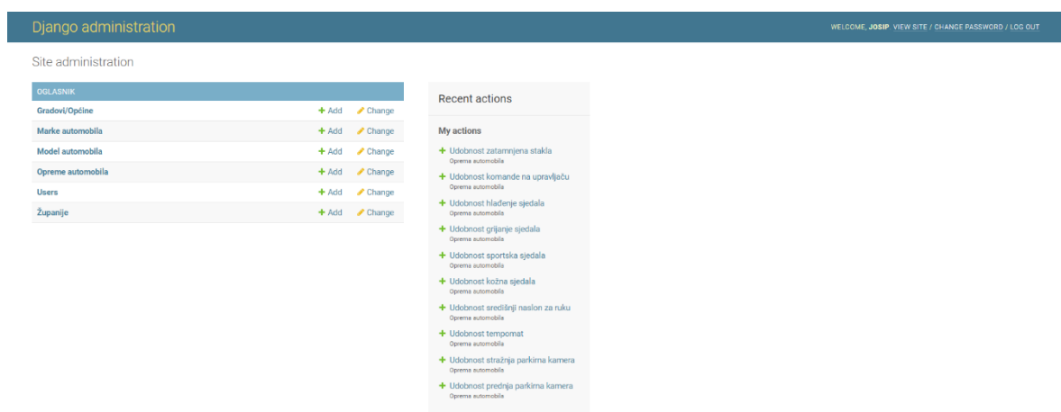
Slika 3: Administratorsko sučelje
