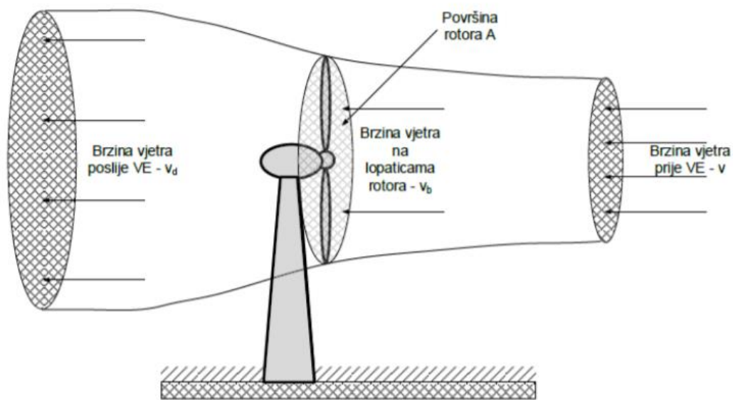
Slika 2.1.- Učinkovitost vjetroturbine [8]
