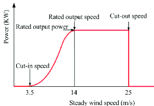
Slika 2.4. Krivulja snage [11]
