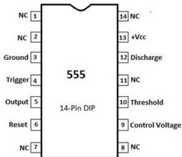
slika 1.2. 16 pinski timer
