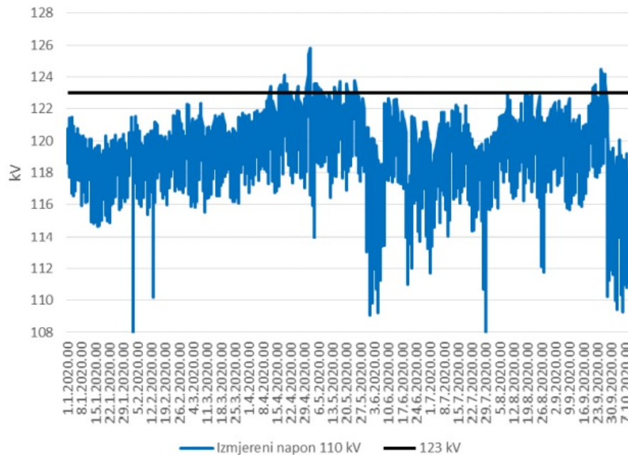
Slika 4.28. Dijagram promjene napona u TS Banja Luka 6 (110 kV) tijekom 2020.
