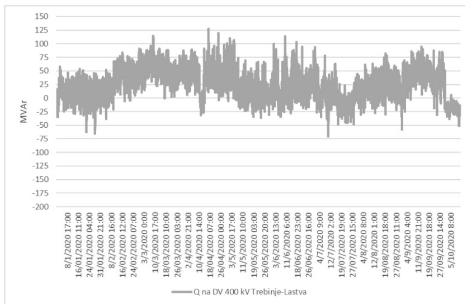
Slika 2. Srednja satna reaktivna snaga na međunarodnom DV 400 kV sa Crnom Gorom
