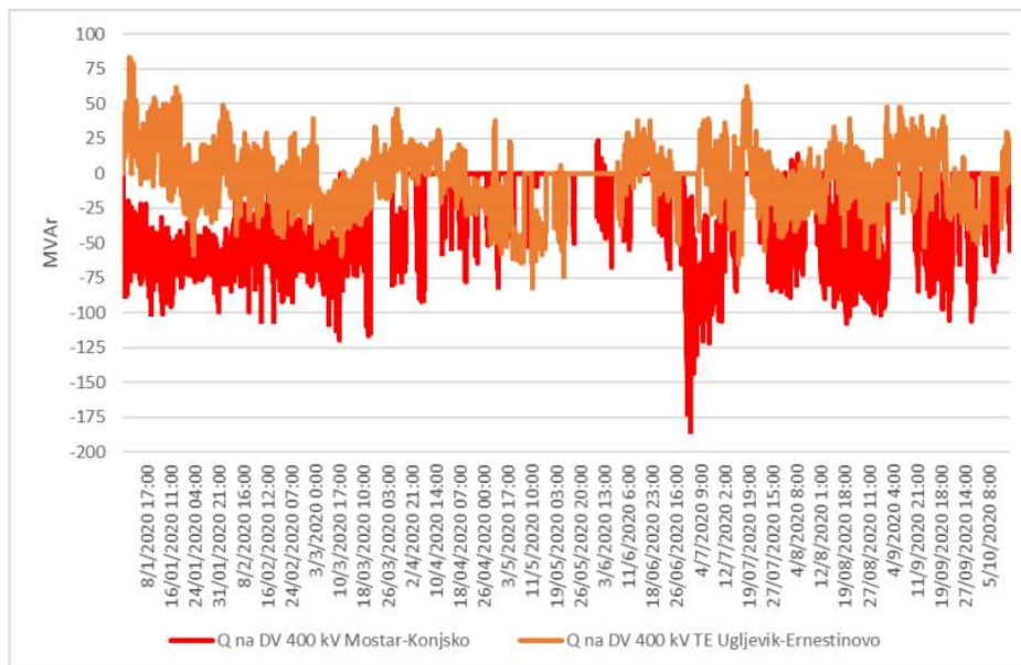
Slika 1. Srednja satna reaktivna snaga na međunarodnom DV 400 kV sa Hrvatskom
