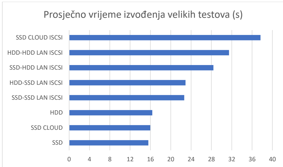
Graf 3: Prosječno vrijeme izvođenja velikih testova na svim obrađenim izvedbama
