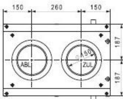
Slika 3.7 - Dimenzije HomeVent FR(201/251/301) uređaja [4]
