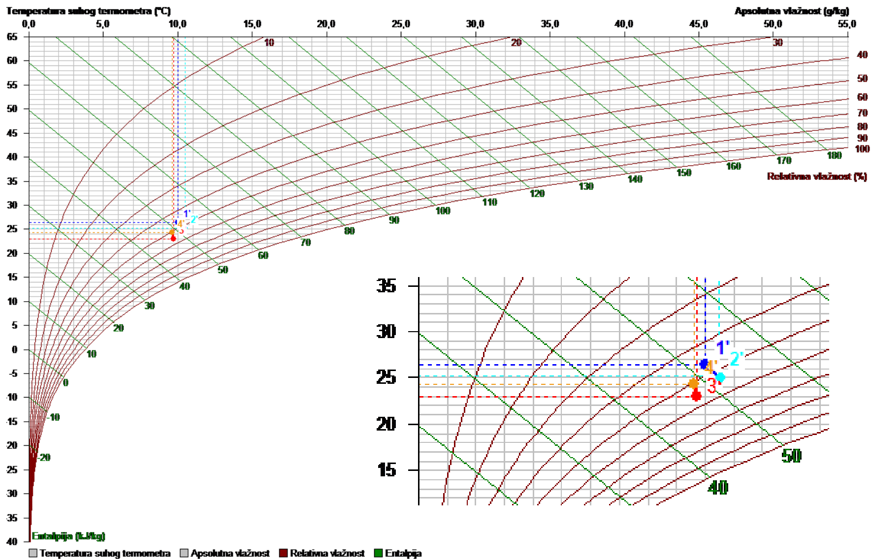
Slika 5.18 - Prikaz druge točke trećeg mjerenja u Mollirovom dijagram [13]
