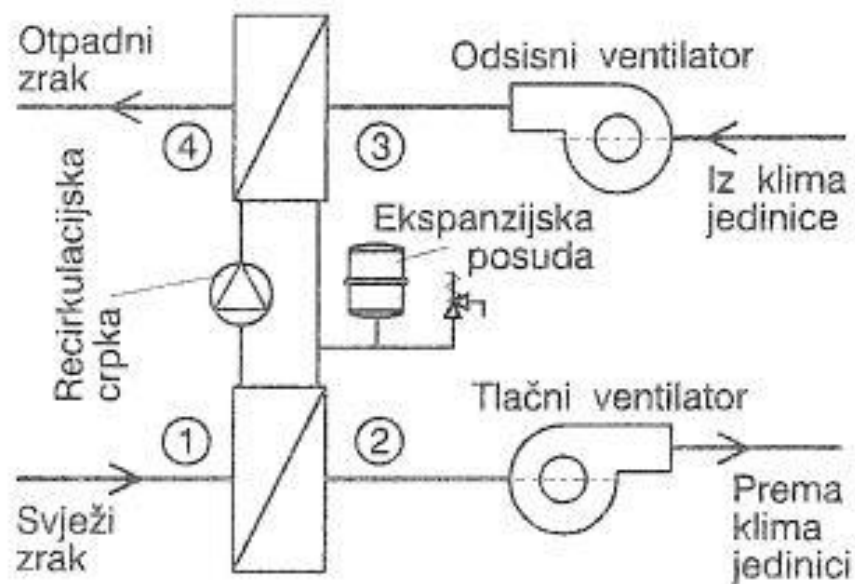
Slika 2.6 - Rekuperator s dva izmjenjivača i posrednim medijem s cirkulacijskom pumpom [9]
