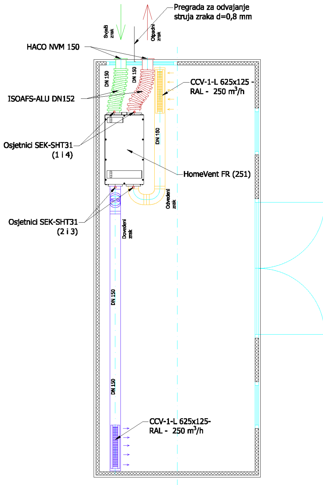
Slika 3.23 - Tlocrt kontejnera s ucrtanom ventilacijom [13]
