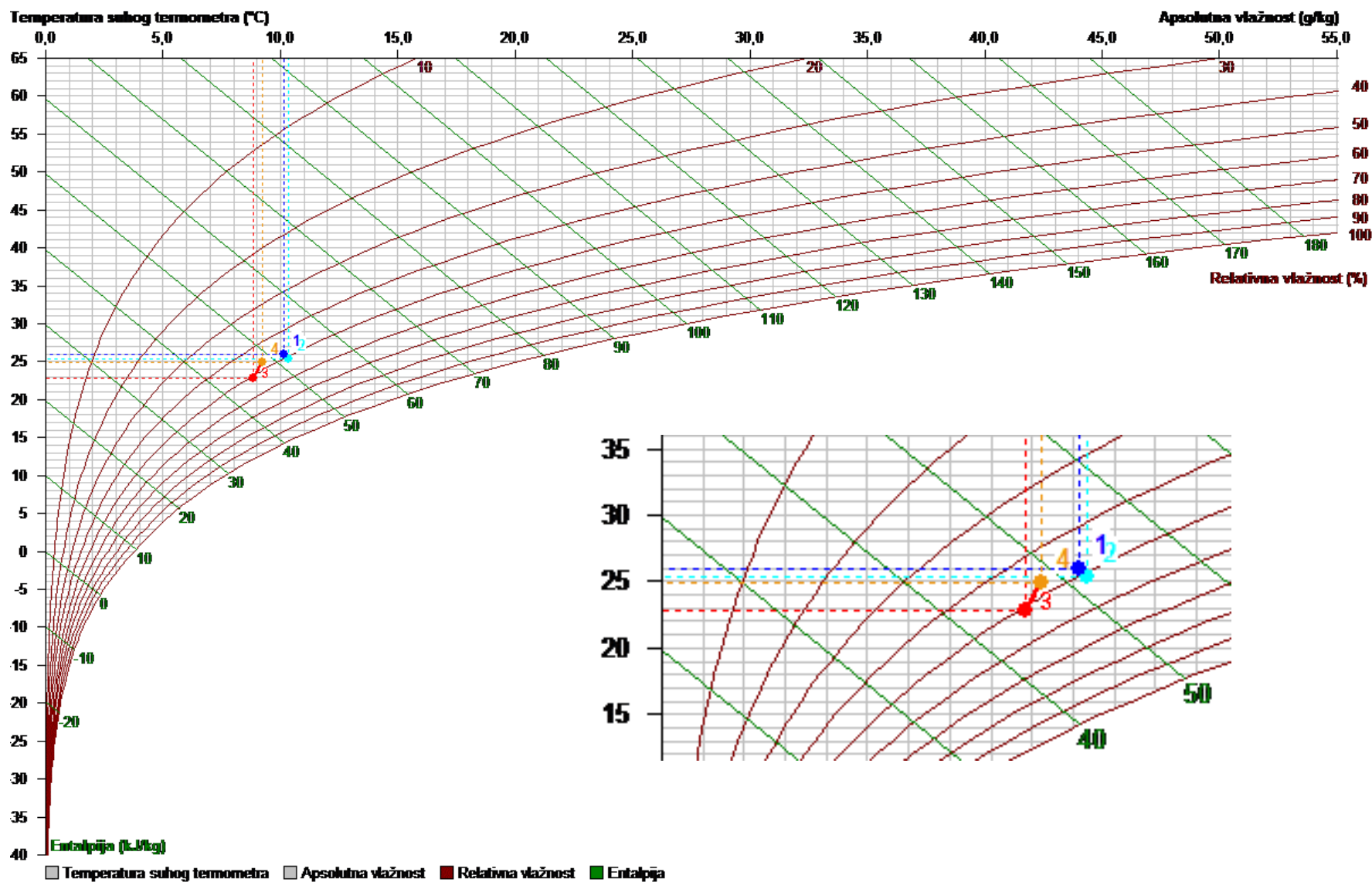
Slika 5.17 - Prikaz prve točke trećeg mjerenja u Molliеровom dijagram [13]
