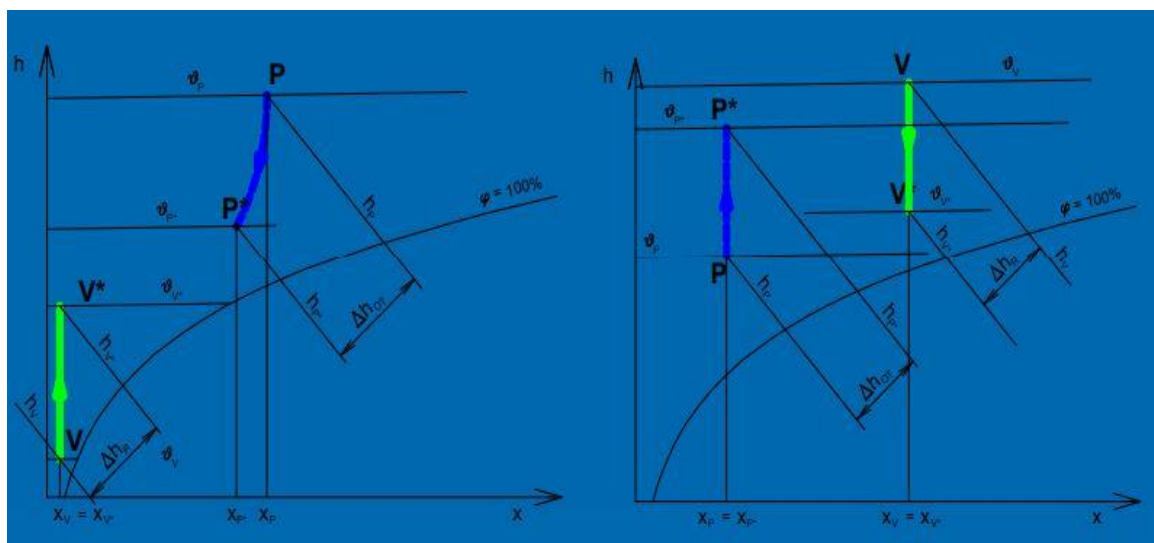
Slika 2.3 - Prikaz povrata toplote u rekuperatoru (lijevo zimi, desno ljeti) [9]
