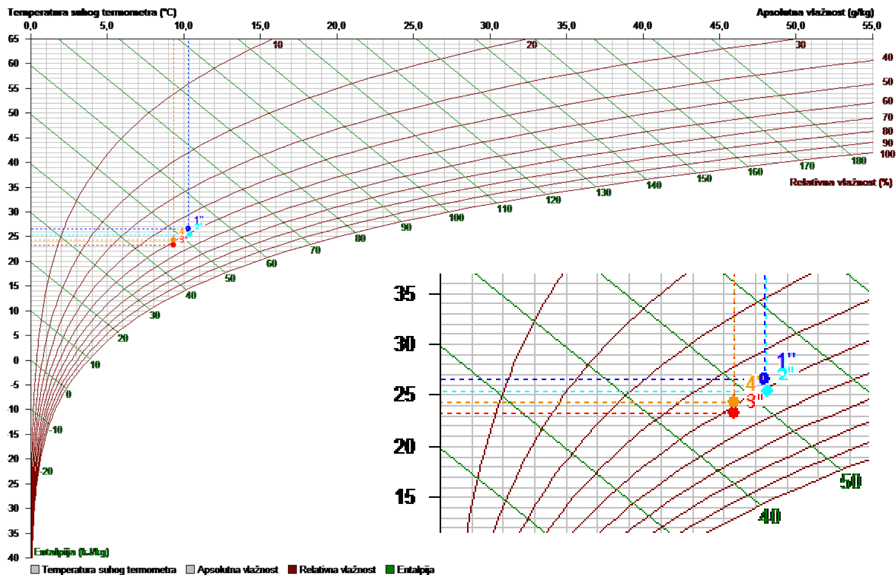
Slika 5.19 - Prikaz treće točke trećeg mjerenja u Mollijevom dijagram [13]
