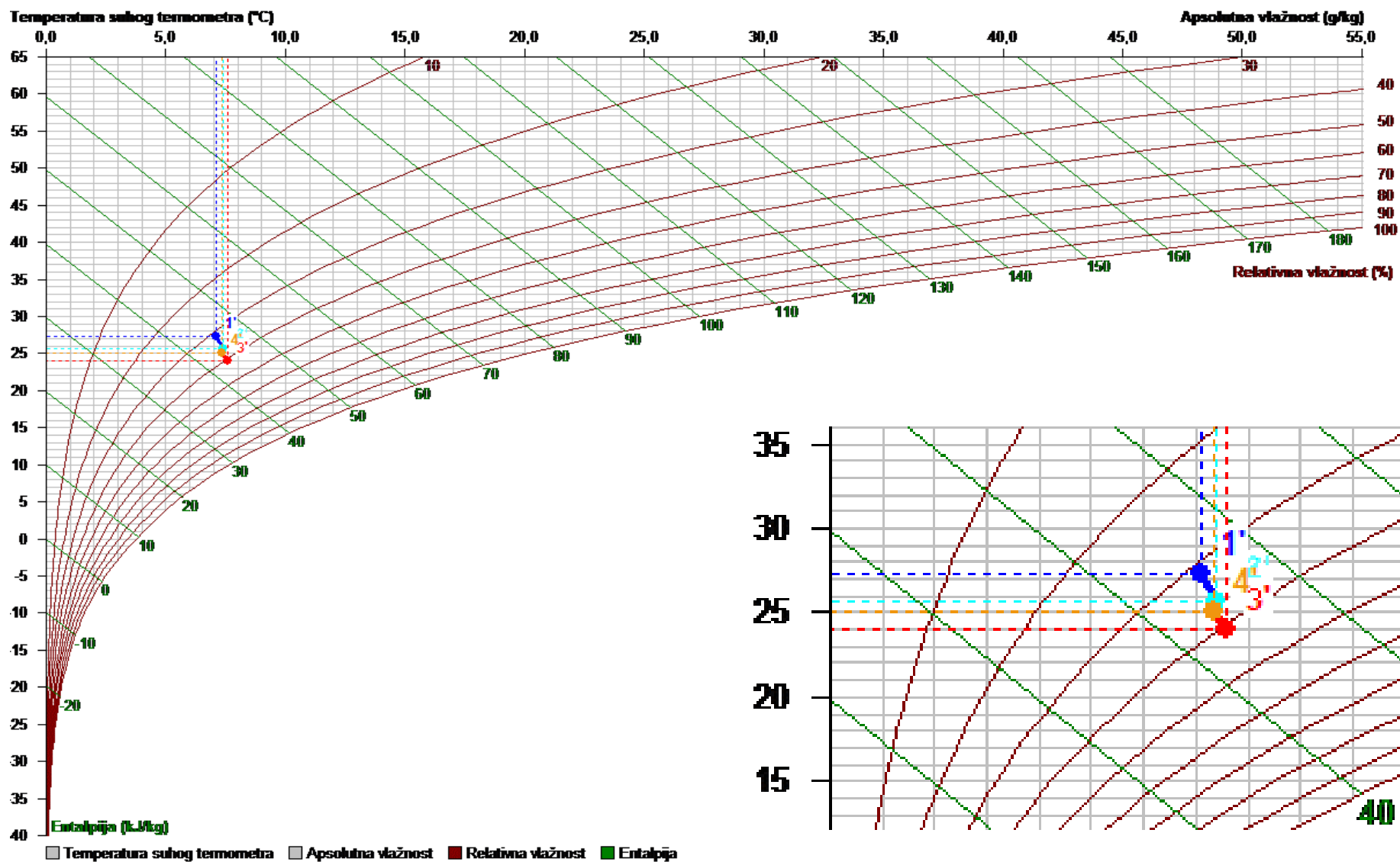
Slika 5.12 - Prikaz druge točke drugog mjerenja u Molliеровom dijagram [13]
