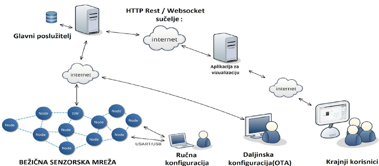
Slika 1. Prikaz bežične senzorske mreže implementirane u Internet Of Things(IOT) koncept
