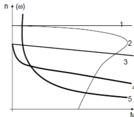
Slika 7. Oblici mehaničkih karakteristika motora. [8]
