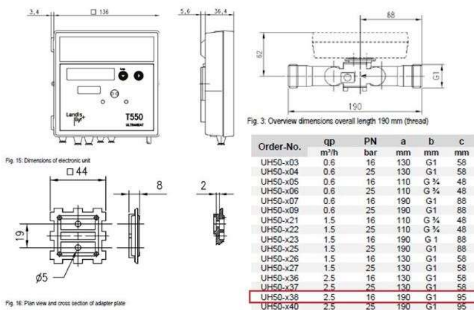
Slika 3.4.2 – Mjerni crtež korištenog mjerača toplinske energije [5]
