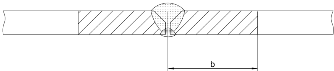
Slika 4.3 Granica zone utjecaja topline
