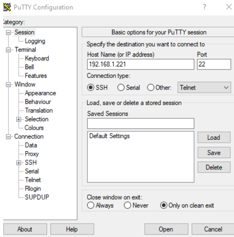
Slika 9.5 Sesijsko sučelje
