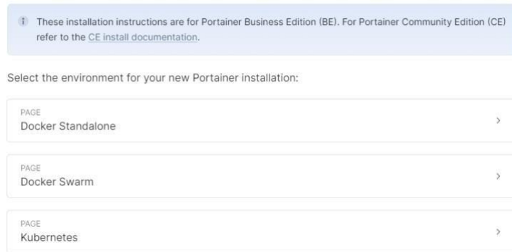
Slika 9.12 Docker verzije
