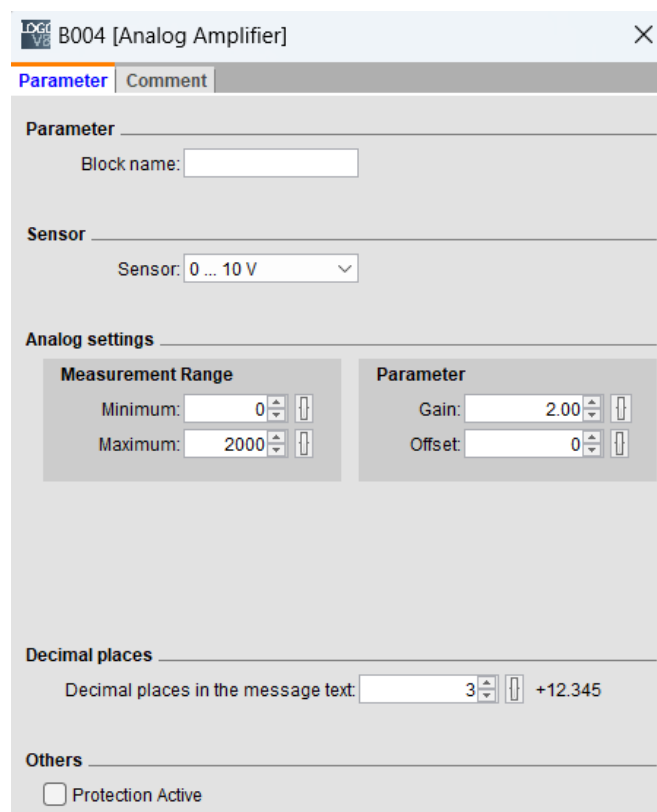
Slika 7.4- Raspon mjerenja tlaka nakon filtera
