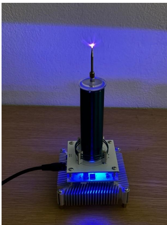
Slika 5. 5: Iskrište zavojnice
