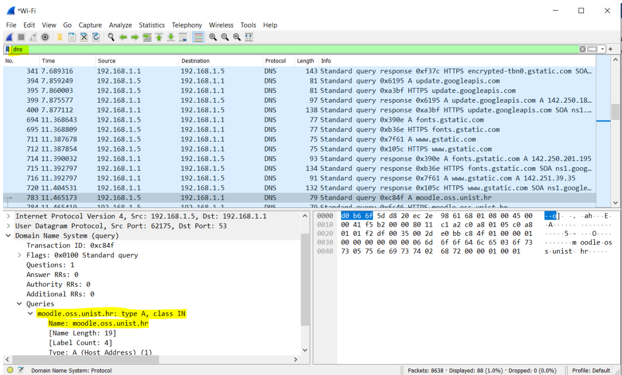
Slika 7 DNS filtriranje
