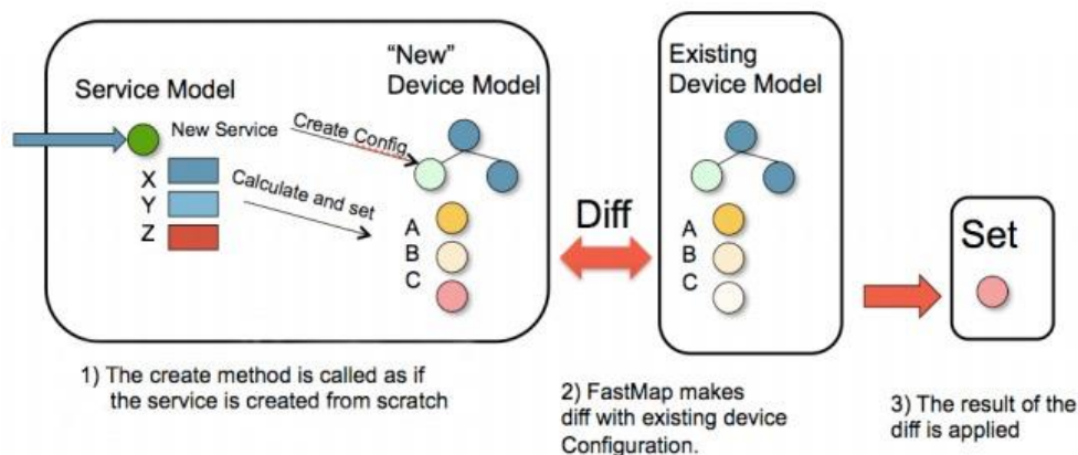
Slika 4.1.1.2. FASTMAP algoritam 31
