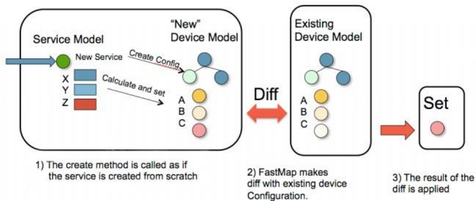
Slika 4.1.1.2. FASTMAP algoritam 31
