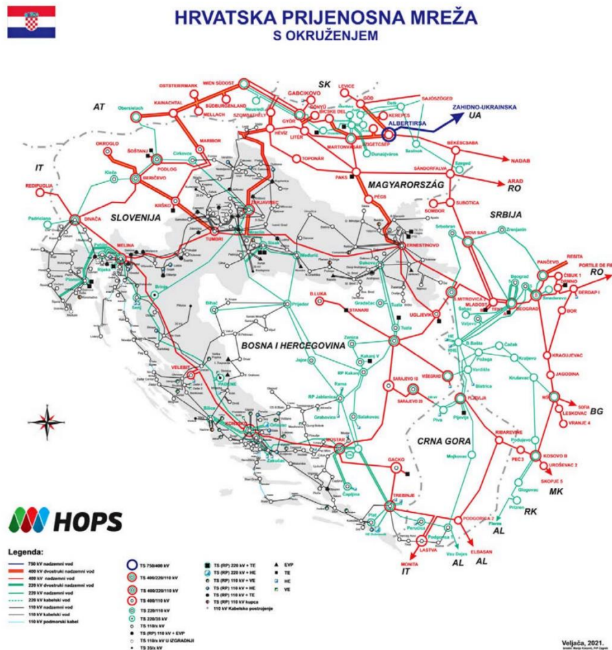
Slika 2.4 Prijenosna mreža s okruženjem [5]
