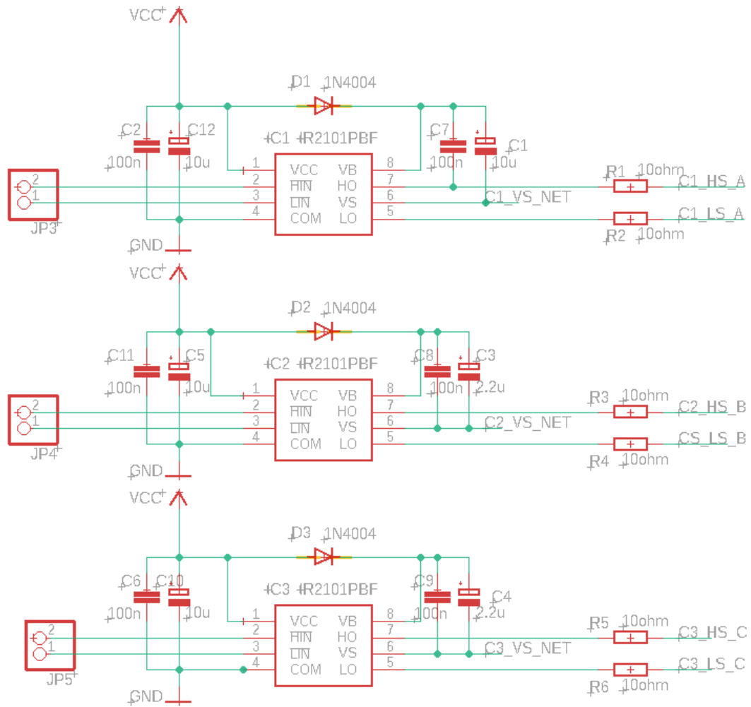
Slika 6.2 Shema spajanja IR2101 mosfet upravljača
