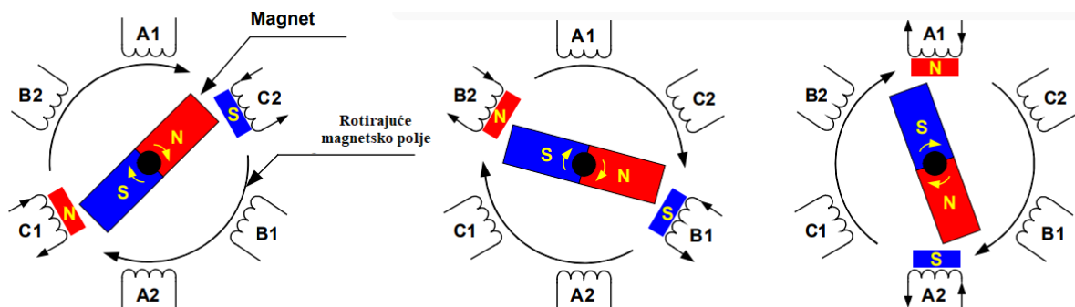
Slika 2.3 Rotacija motora [1]
