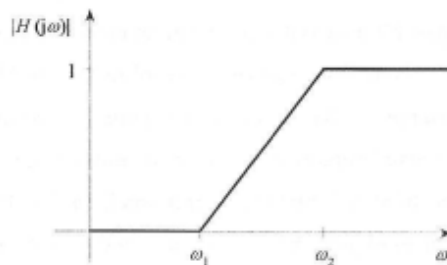
Slika 3.2. Frekvencijska karakteristika visoko propusnog filtra
