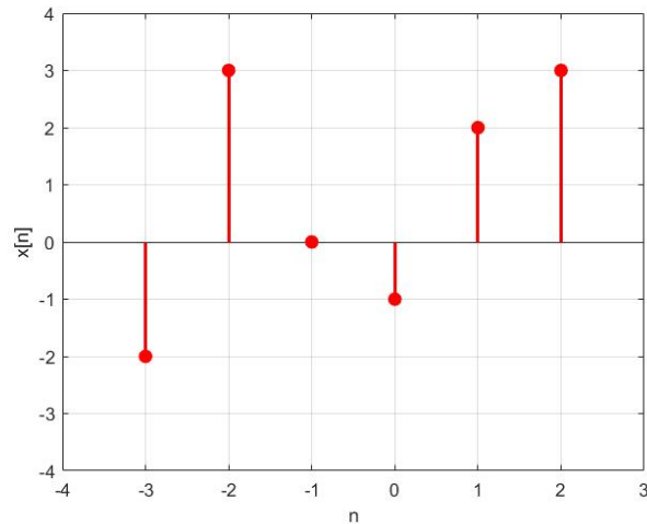
Slika 2.2. Diskretni signal
