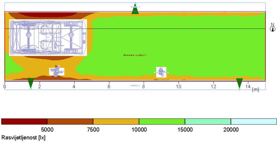
Slika 3.38. Rasvjetljenost prilaza i položaj senzora
