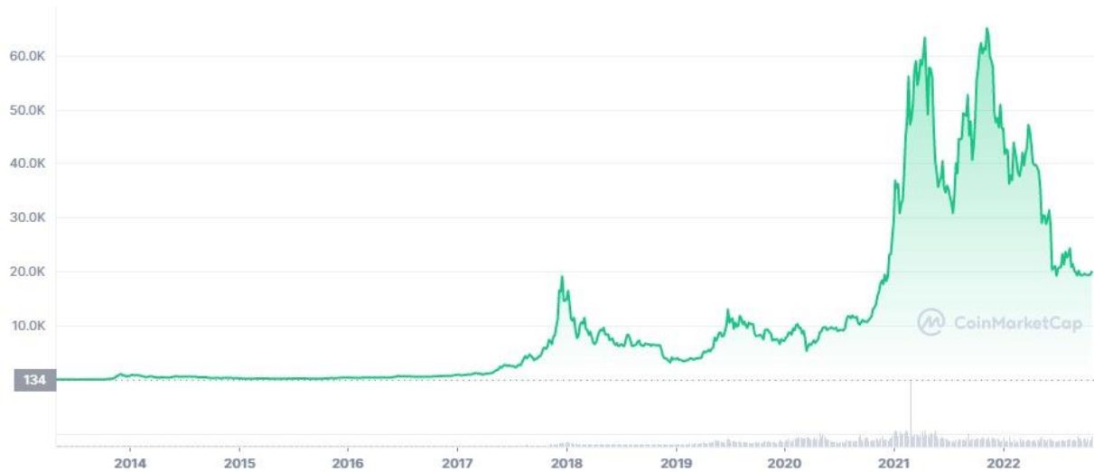
Slika 4.6 Grafički prikaz cijene bitcoina izražene u dolarima (2013-2022)
