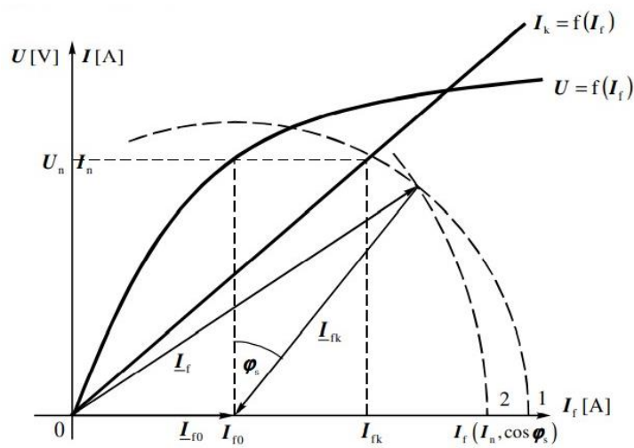
Slika 2.10. Švedski dijagram [1]
