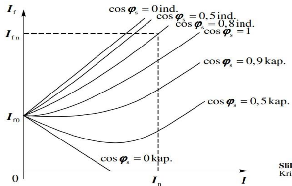
Slika 2.9. Krivulje regulacije [1]
